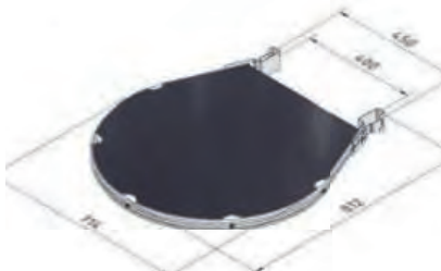
Plataforma fija
