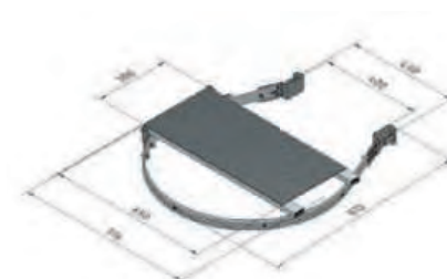
Puerta de seguridad para acceso / Plataforma intermedia abatible
